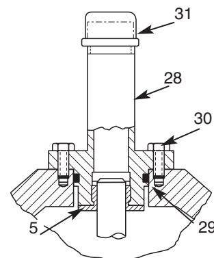
DETALLE DE LA TAPA DE 16"
